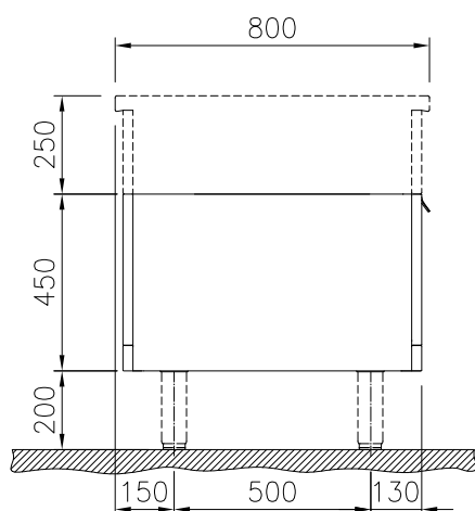
Zij aanzicht
